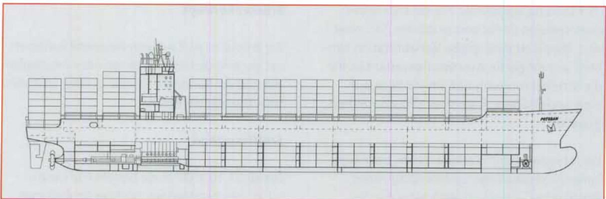
Seitenansicht des MS "Potsdam"
